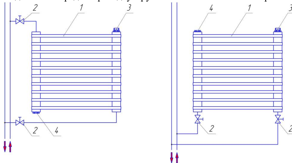
Рис. 3 1. Радиатор. 2. Вентиль (кран). 3. Кран Маевского-воздухоотводчик. 4. Пробка глухая.
