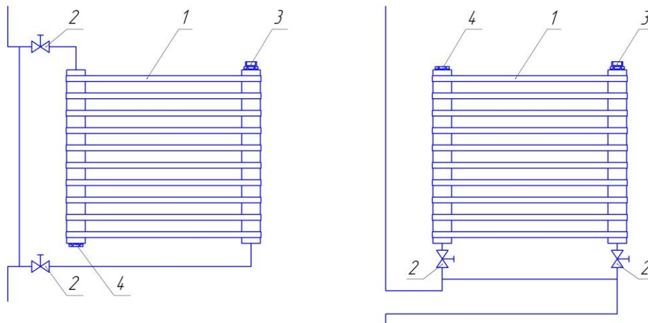
Рис.2 1. Радиатор. 2. Вентиль (кран). 3. Кран Маевского-воздухоотводчик. 4. Пробка глухая.
